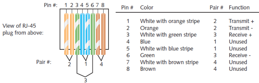
Gambar 5. Kabel UTP dengan standar 568B
