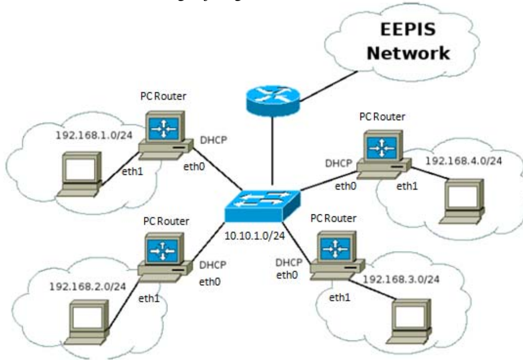
Gambar 3. Konfigurasi jaringan untuk Dynamic Routing
